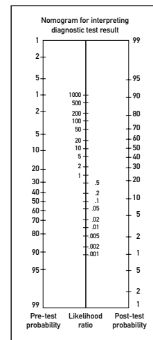
Abbildung 2: Das Fagan-Nomogramm
